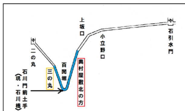
図-1 辰巳用水建設当初の管路部の簡略縦断面
